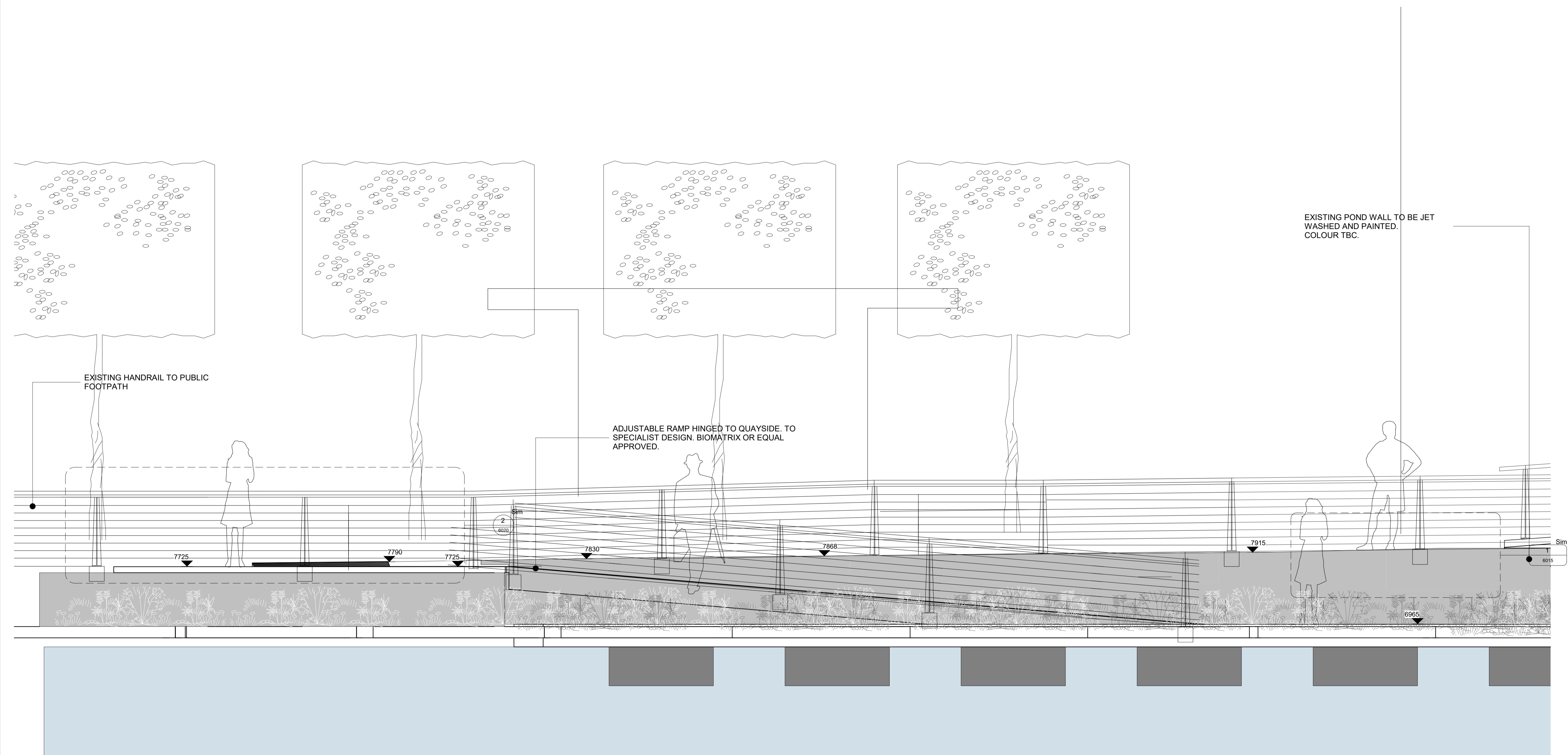
Section 9 1:25
